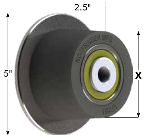
3.5" UR/STL 107591 4" UR/STL 107594
