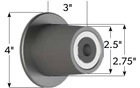
H.T. STEEL 107628
